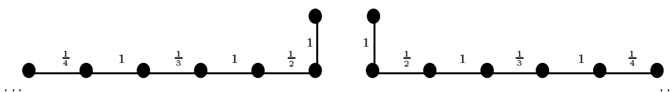
Abbildung 2.7: Graphen dieser Form sollen an den Graphen aus Abbildung 2.6 so angefügt werden, daß die beiden Zusammenhangskomponenten durch eine Kante mit Gewicht Eins überbrückt werden.
