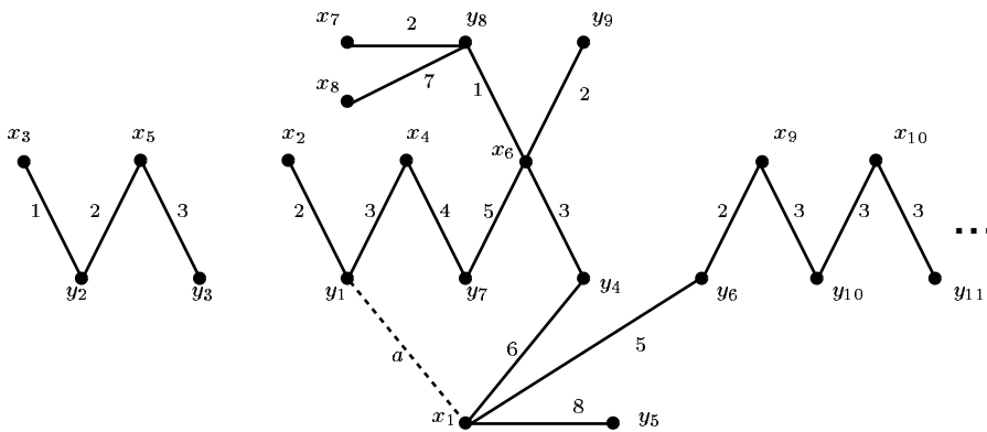
Abbildung 2.2: G(P_a)
