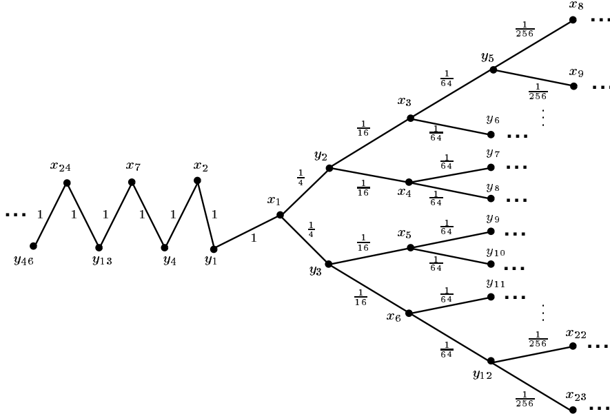
Abbildung 2.4: G(P)
