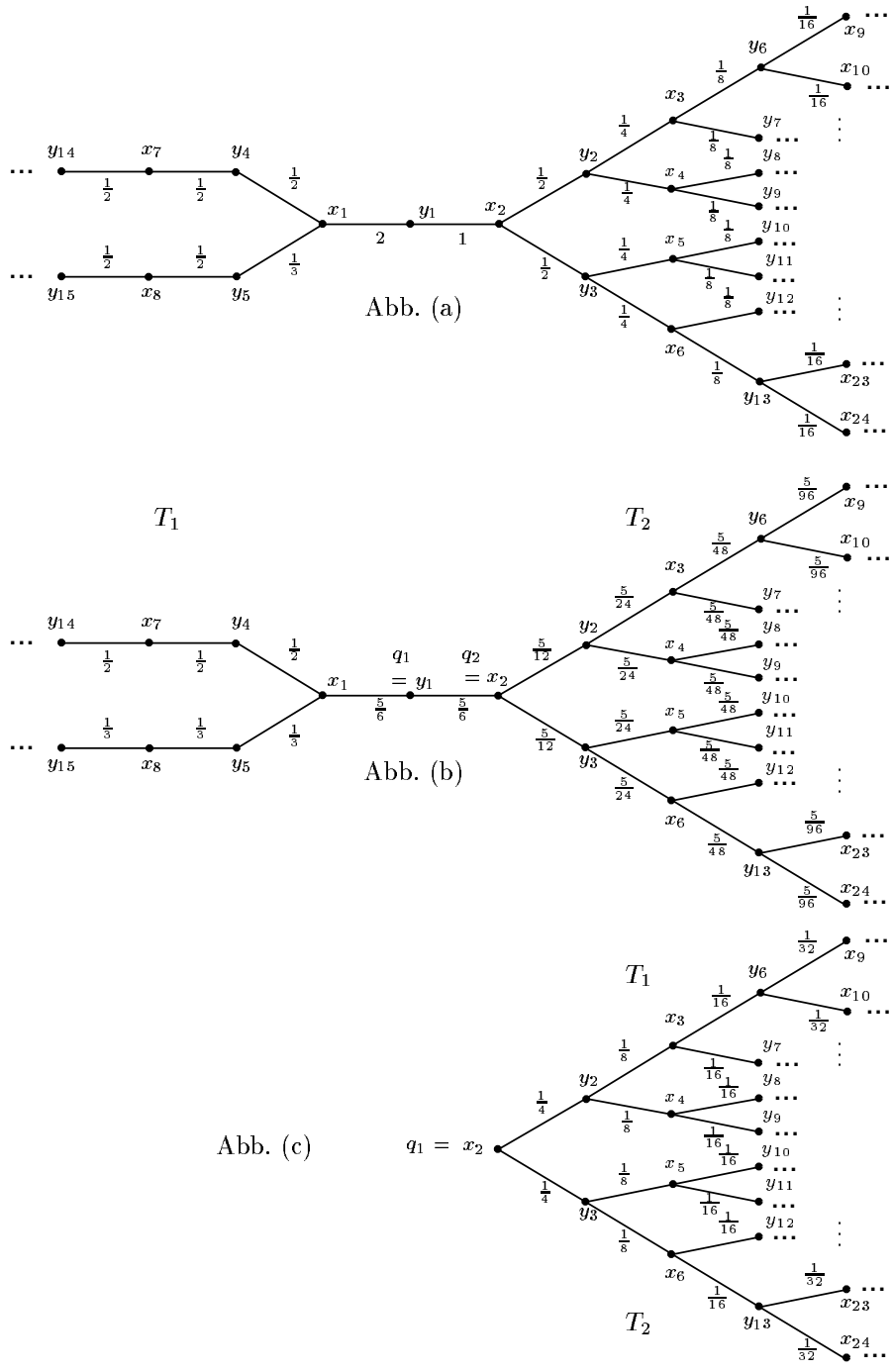
Abbildung 2.3: G(P) (in (a)) und zwei Teilgraphen H_1 \leq G(P) (in (b)), H_2 \leq G(P) (in (c))
