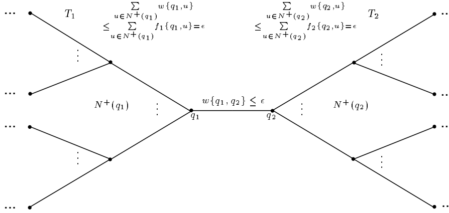
Abbildung 2.1: \epsilon -Doppelbaum
