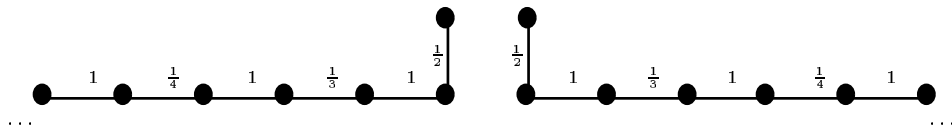
Abbildung 2.8: Graphen dieser Form sollen an den Graphen aus Abbildung 2.6 so angefügt werden, daß die beiden Zusammenhangskomponenten durch eine Kante mit Gewicht \frac{1}{n} überbrückt werden.
