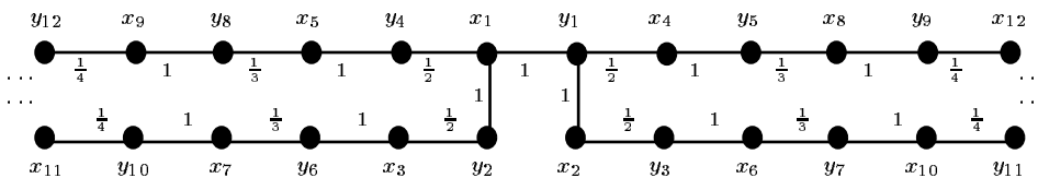
Abbildung 2.6: Der Graph soll, wie angedeutet, nach links und rechts ins Unendliche fortgesetzt werden. Das Bildungsgesetz für die Ecken ist dabei links oben \dots, y_{4(n+1)}, x_{4n+1}, \dots , links unten \dots, x_{4n+3}, y_{4n+2}, \dots , rechts oben \dots, y_{4n+1}, x_{4(n+1)}, \dots , rechts unten \dots, x_{4n+2}, y_{4n+3}, \dots
